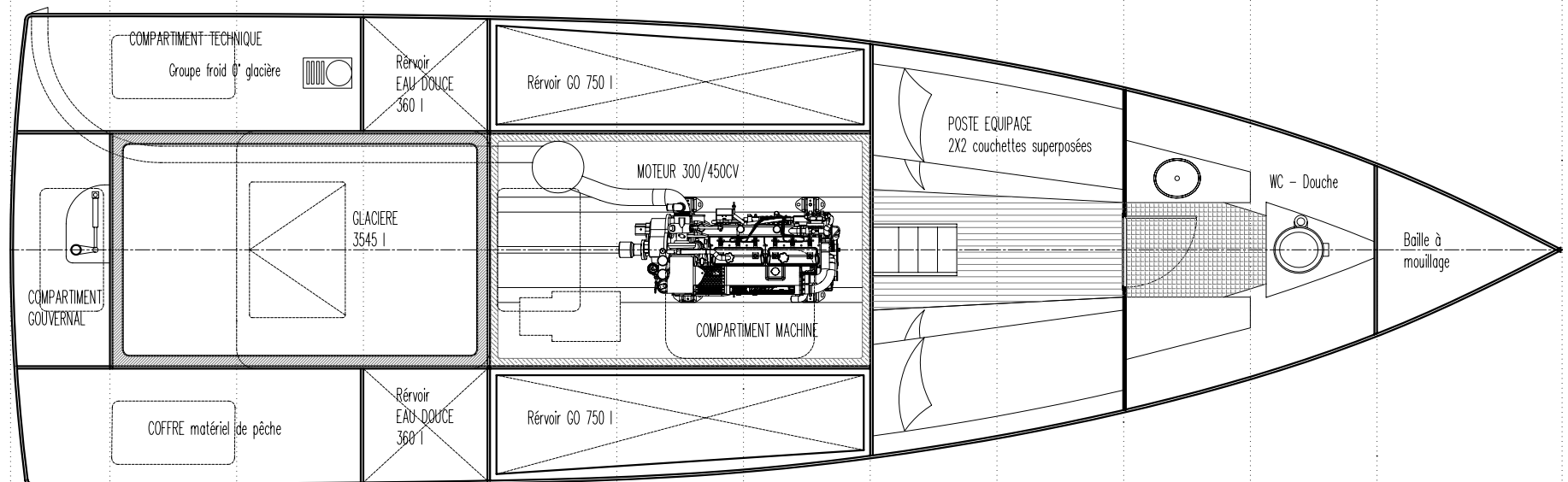
PLAN DE SOUTE
