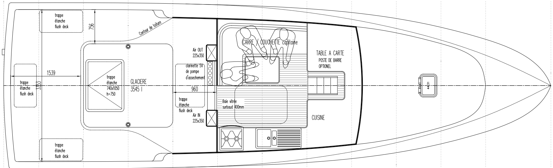
PLAN DE PONT
